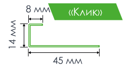
Соединительный профиль
