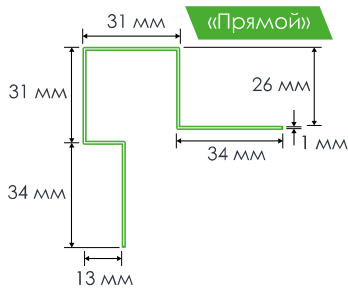
Внешний асимметричный угловой профиль
