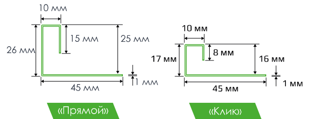
Конечный профиль
