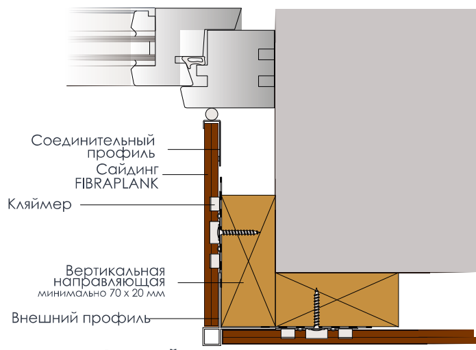
Внешний асимметричный угловой профиль
